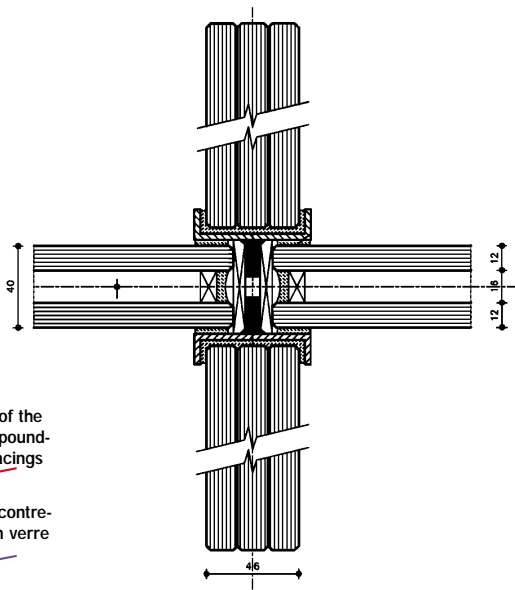
Detailzeichnung der Windversteifungen aus dreischichtigem Glas
